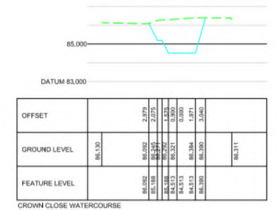
CROWN CLOSE WATERCOURSE CHAINAGE 10.000
